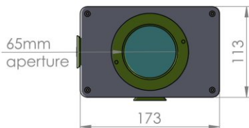
3" Front Lid
