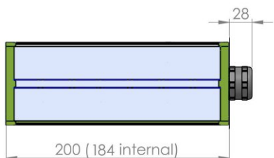
Rückwand C
